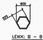
LEIKK. B - B
