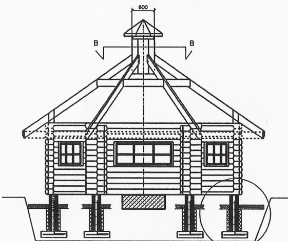
HUOM: HIRSIKEHIÄ EI OLE LEIKATTU LEIKK. A - A
